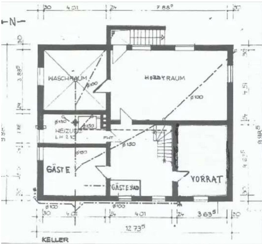
UG Grundriss
